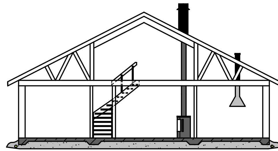
Sektionsritning
